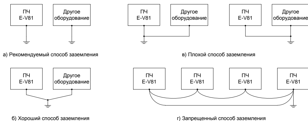
Рисунок 5-6 – Способы заземления
