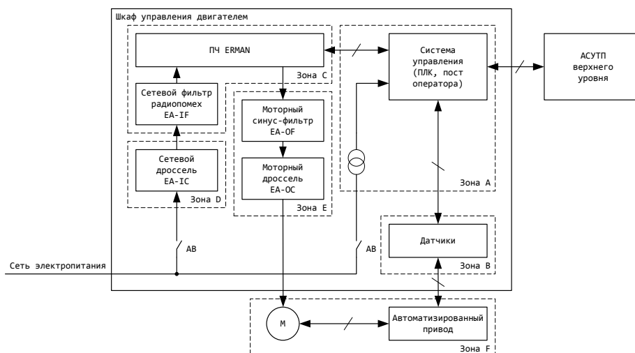
Рисунок 5-30 – Размещение устройств автоматизации в шкафу
