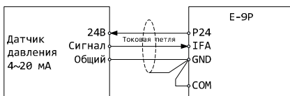
Схема подключения датчика давления с токовым выходом 4-20 мА
