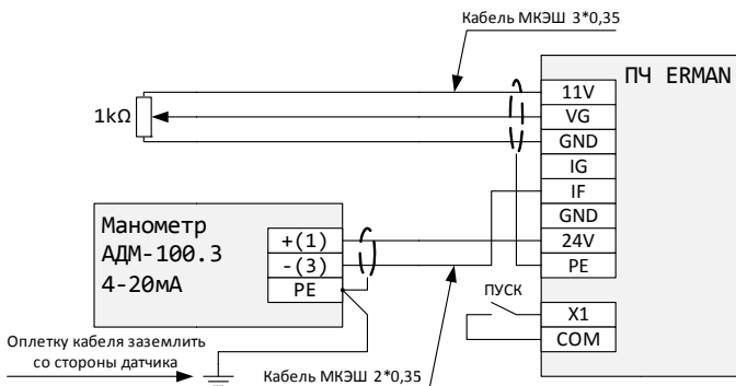
Рисунок 18 – Подключение манометра АДМ-100.3 и потенциометра задания уставки
