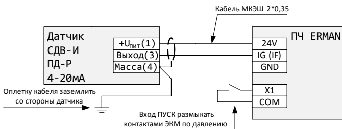
Рисунок 16 – Подключение датчиков давления типа СДВ-И, ПД-Р и т.п.
