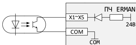
Рисунок 12 – Подключение сигнала типа «открытый коллектор»
