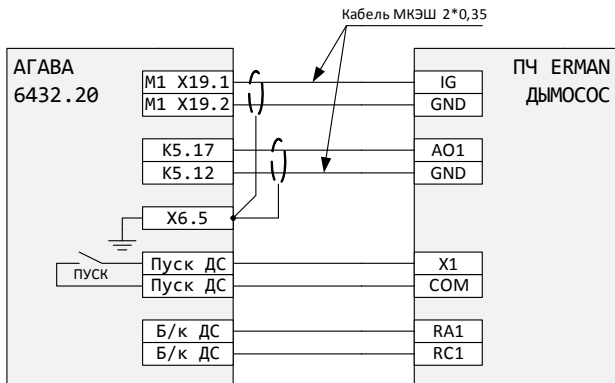
Рисунок 20 – Подключение к шкафу котловой автоматики АГАВА 6432.20 (дымосос)
