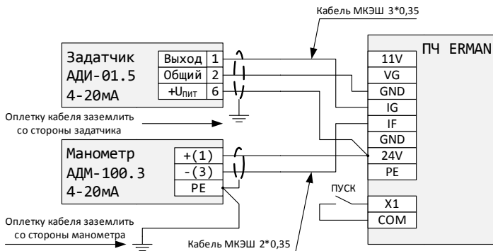
Рисунок 19 – Подключение манометра АДМ-100.3 и цифрового задатчика уставки АДИ-01.5
