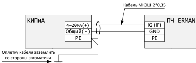
Рисунок 14 – Подключение сигнала типа «4-20 мА» или «0-20 мА»
