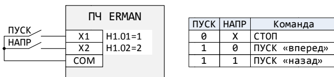
Рисунок 29 – Двухпроводная схема управления (дополнительный провод используется для переключения направления)
