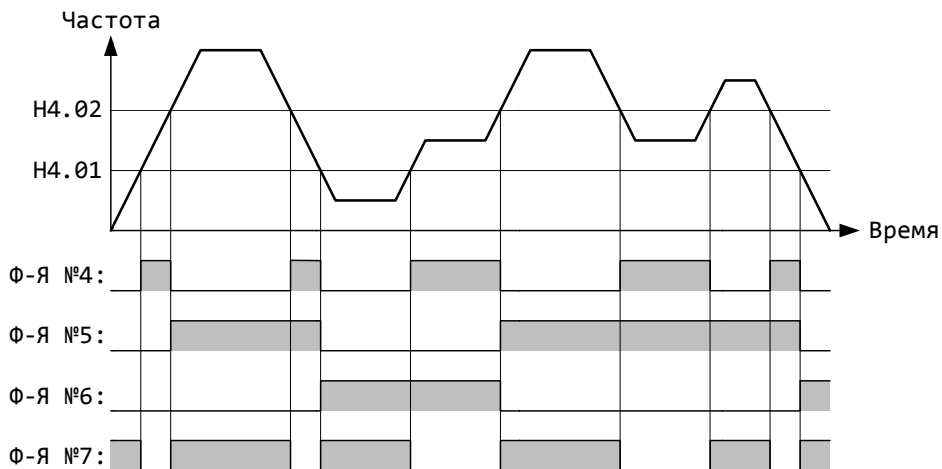
Рисунок 32 –Функции релейных выходов №4, №5, №6, №7
