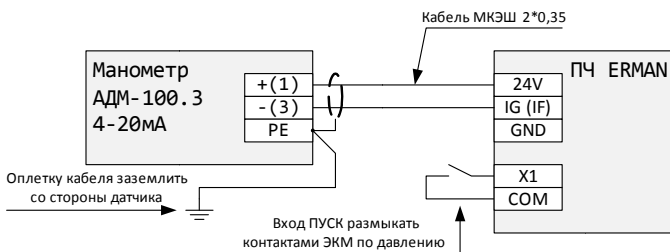
Рисунок 15 – Подключение электронного манометра АДМ-100.3
