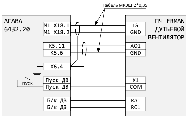
Рисунок 21 – Подключение к шкафу котловой автоматики АГАВА 6432.20 (вентилятор)
