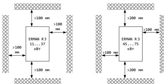
Рисунок 6 – Воздушные зазоры для установки ПЧ, не менее
