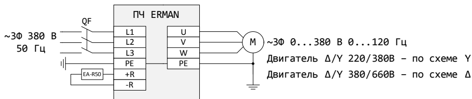
Рисунок 8 – Подключение ПЧ 7,5...37 кВт 380 В с тормозным резистором EA-R50 (опция)
