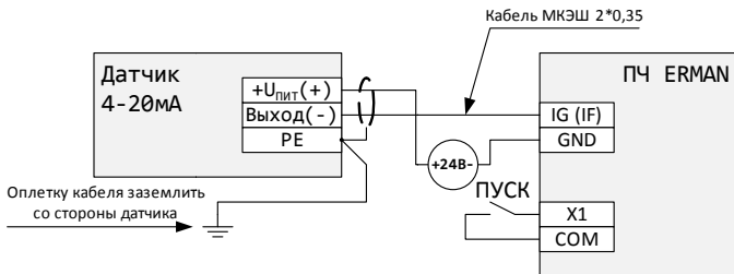
Рисунок 17 – Подключение датчика с внешним питанием
