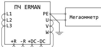
Рисунок 33 – Испытание сопротивления изоляции
