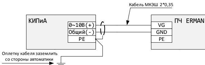
Рисунок 13 – Подключение сигнала типа «0-10 В» или «0-5 В»
