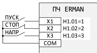
Рисунок 30 – Трехпроводная схема управления
