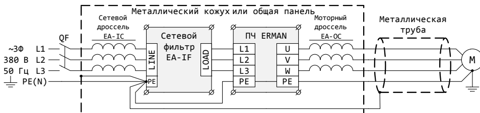
Рисунок 24 – Снижение уровня высокочастотных помех
