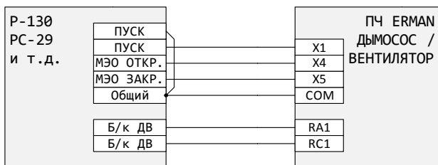
Рисунок 22 – Подключение к позиционным регуляторам "Больше/Меньше" вместо МЭО (при необходимости используйте промежуточные реле для развязки)
