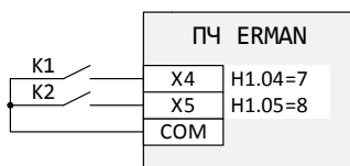
Рисунок 31 – Выбор частоты / уставки с помощью входов СКОРОСТЬ 1, СКОРОСТЬ 2
