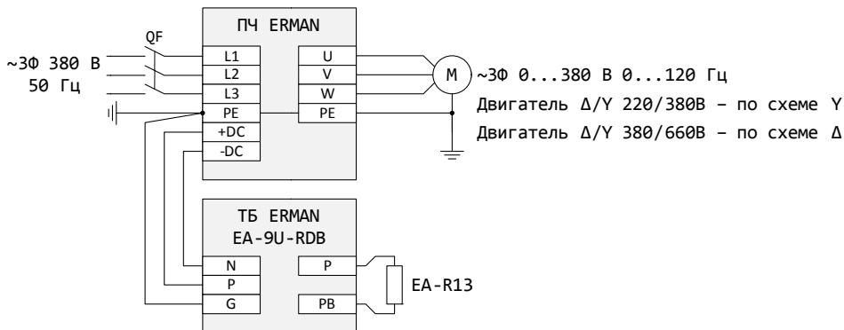
Рисунок 9 – Подключение ПЧ 45...93 кВт 380 В с тормозным резистором и внешним тормозным блоком (опция)
