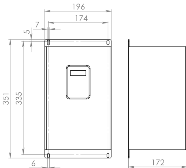
Рисунок 3 – размеры ПЧ мощностью от 7,5 до 15 кВт
