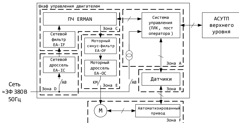
Рисунок 23 – Способ размещения устройств автоматизации в шкафу
